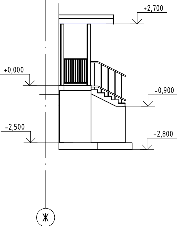
Фрагмент фасада м 1:100
