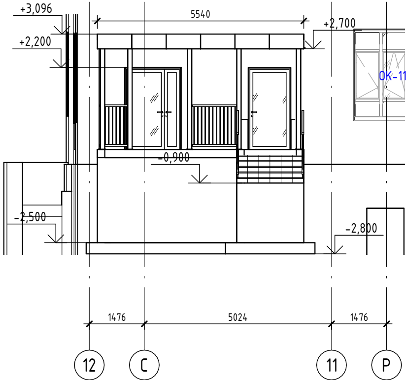
Фрагмент фасада м 1:100
